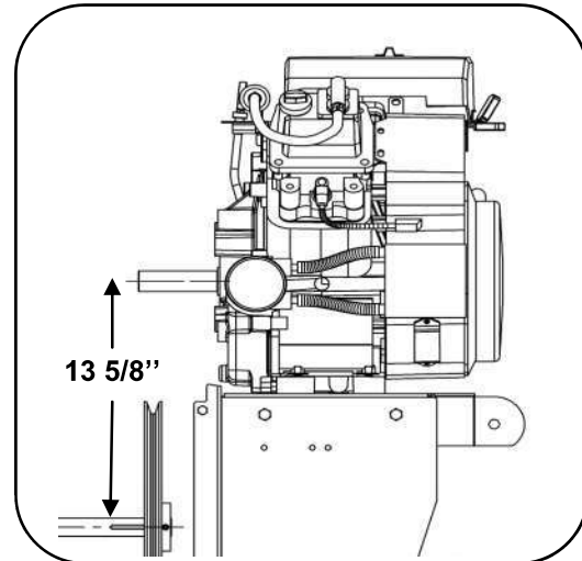
Vérification de la hauteur du moteur
