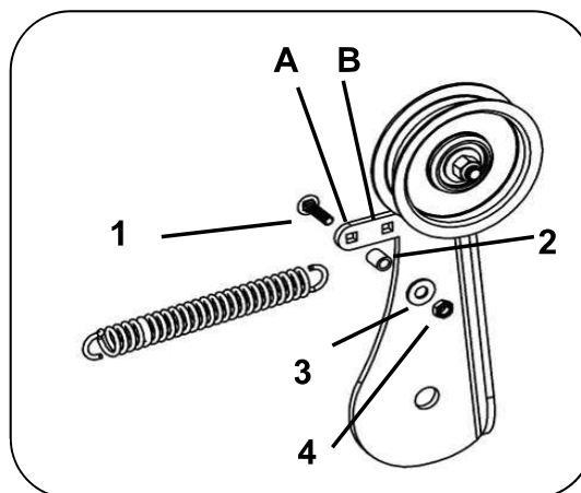
Ajustement de la tension de la courroie
