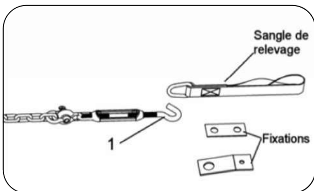
Installation des tendeurs sur le véhicule
