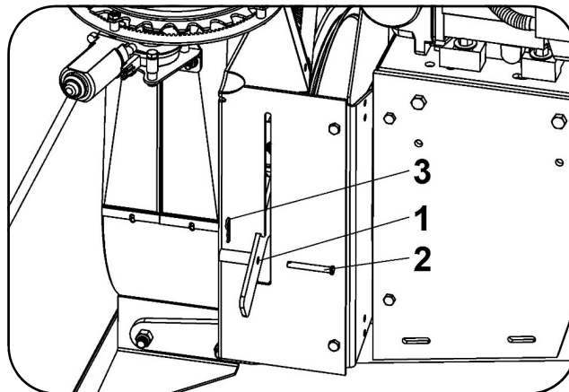
Sécuriser le tensionneur
