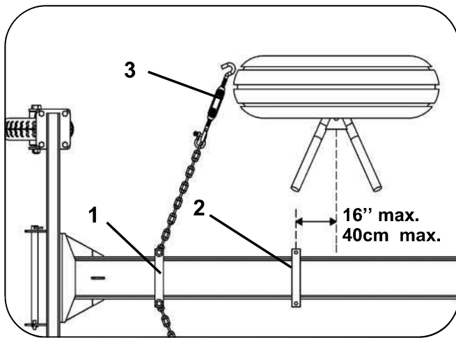
Vérification de l'installation des tendeurs
