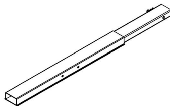
EXTENSION DU SOUS-CHÂSSIS #700485 Pour les véhicules plus long.
