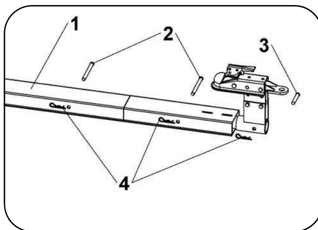
Fixation du sous-châssis
