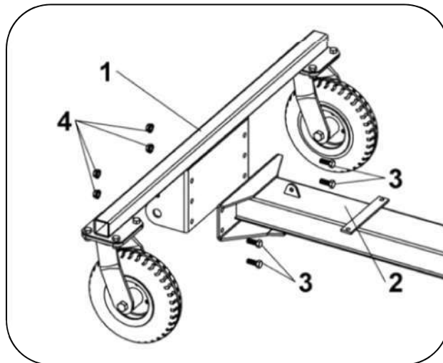
Installation du support de roue
